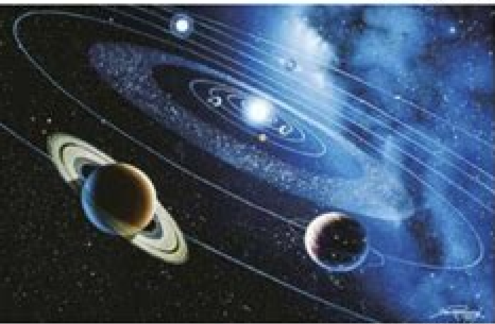
Representación actual del sistema solar
